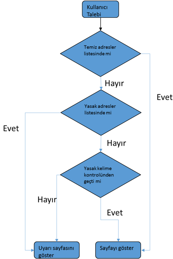
Şekil 3.5 Filtreleme Algoritması
