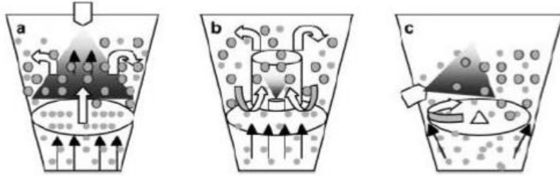
Şekil 2.13 Yukarıdan (a), aşağıdan (b) ve teğetsel püskürtmeli (c) akışkan yatak yöntemleri ile mikrokapsülasyonun şematik gösterimi (Ghosh 2006).
