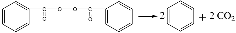
Şekil 2.2 Benzoilperoksit(BPO) başlatıcısının parçalanma reaksiyonu.
