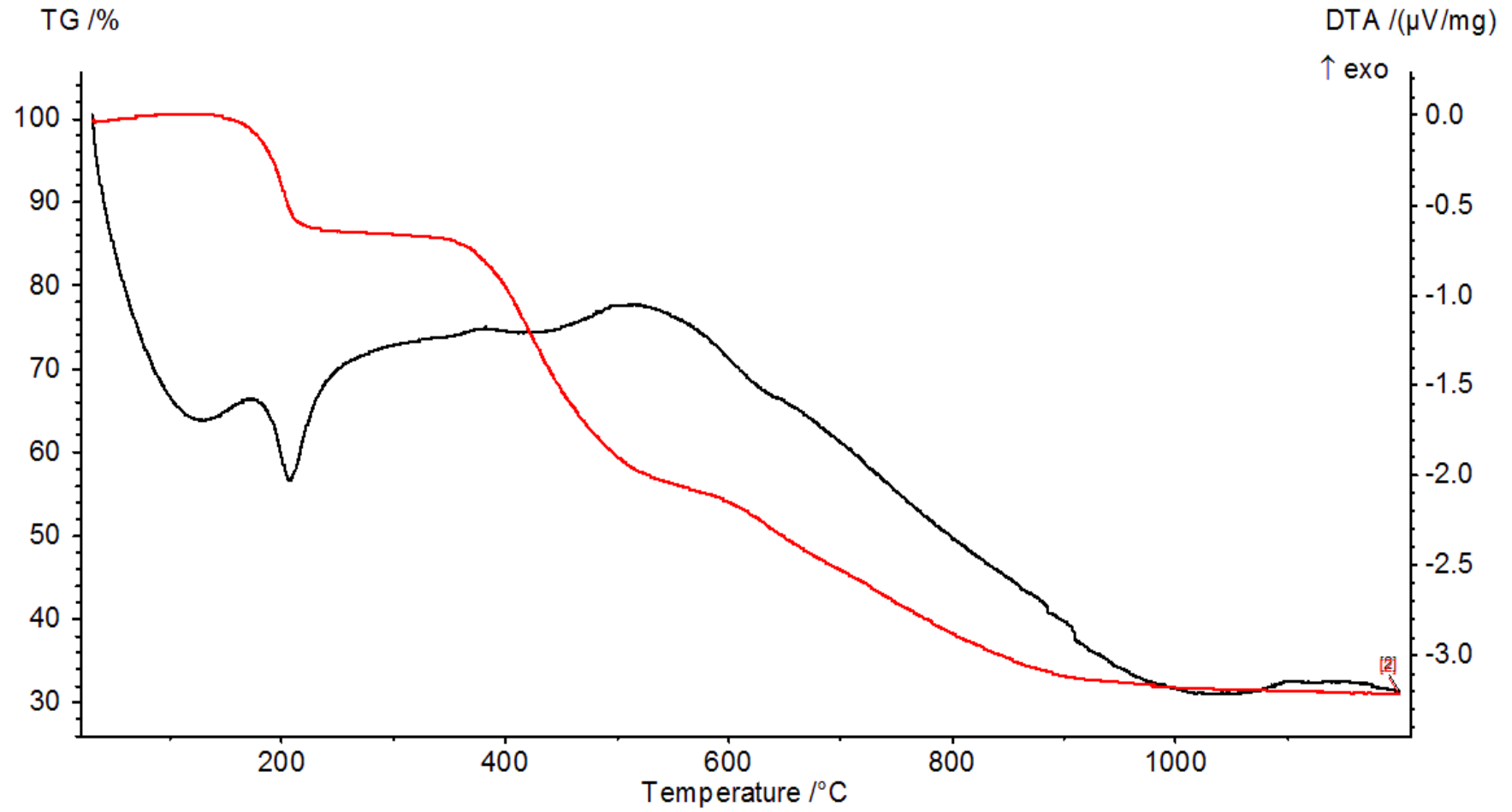
Şekil 4.8 Vanadyum ve piridin-2,6-karboksilato ligandı içeren yeşil renkli koordinasyon bileşiğin TGA ve DTA eğrileri.
