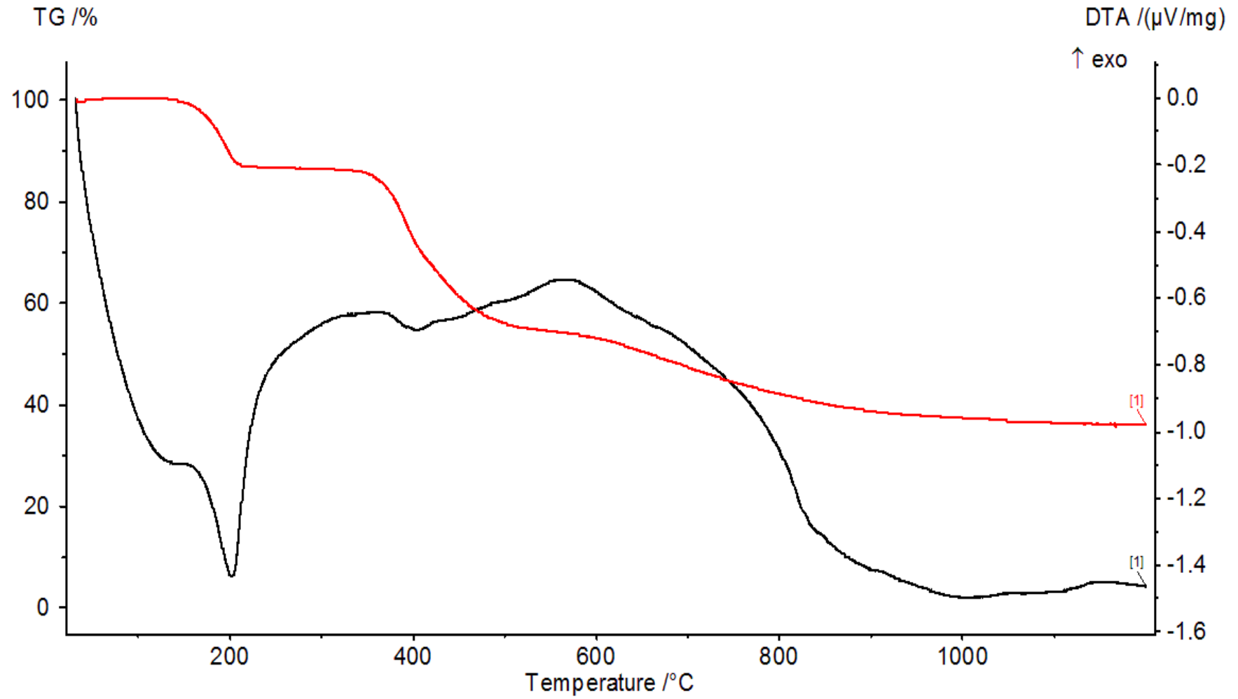
Şekil 4.4 Vanadyum ve piridin-2,6-karboksilato ligandı içeren sarı renkli koordinasyon bileşiğın TGA ve DTA eğrileri.
