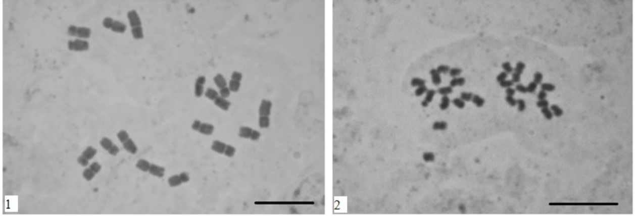
Şekil 1. Metafaz kromozomları; 1- C. fenzlii 2- O. acutidens Scala bar 10 \mu\text{m} .
