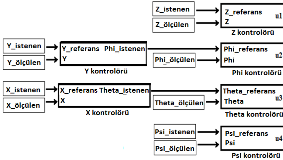
Şekil 3.17 Dört rotorlu İHA'nın kontrolör yapısı.
