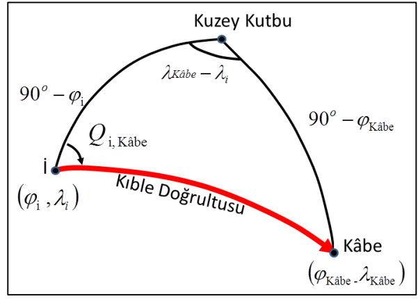
Şekil 3. Küresel üçgen üzerinde kible açısı
