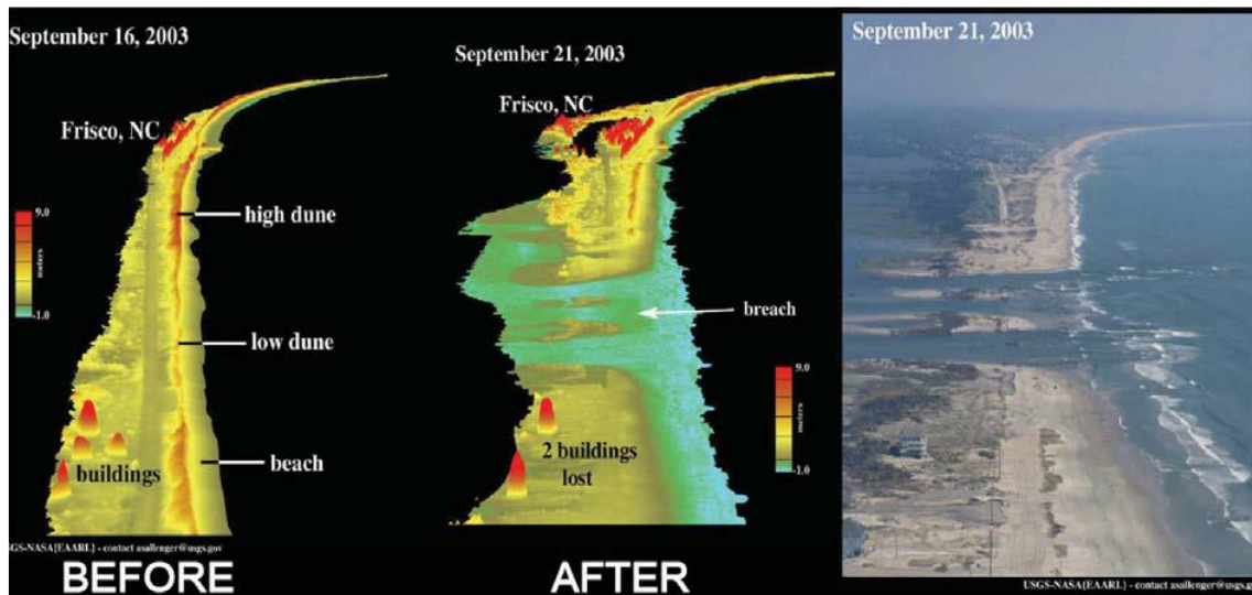
Resim 3.1 LIDAR uygulaması (Uzel 2013).
