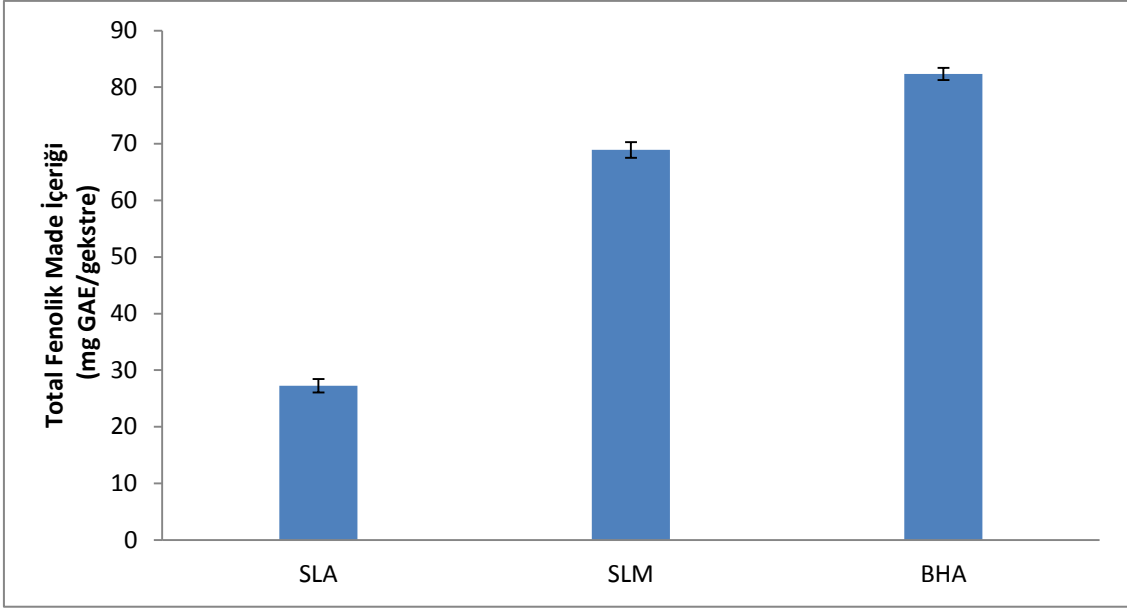
Şekil 4.3 Stachys tmolea Boiss. bitkisinin metanol ve aseton ekstraları ile standart antioksidan maddelerin total fenolik madde içeriği.
