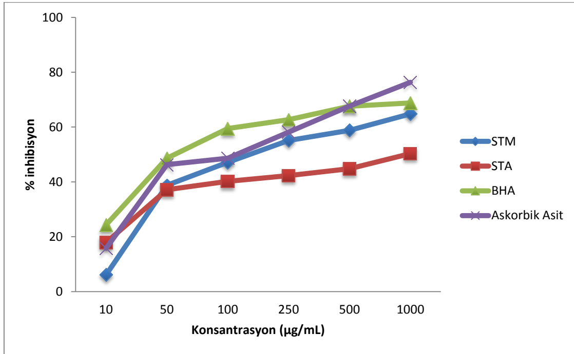
Şekil 4.1 Stachys tmolea Boiss. Bitkisinin metanol ve aseton ekstraları ile standart maddelerin % inhibisyon değerleri.
