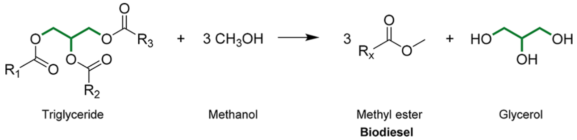
Şekil 1.3 Yağlardan biyodizel ve gliserol oluşumu (Dodekatos vd. 2018a).
