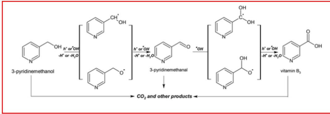
Şekil 1.5 3-Piridinmetanolün fotokatalitik yükseltgenme mekanizması (Yurdakal vd. 2017).
