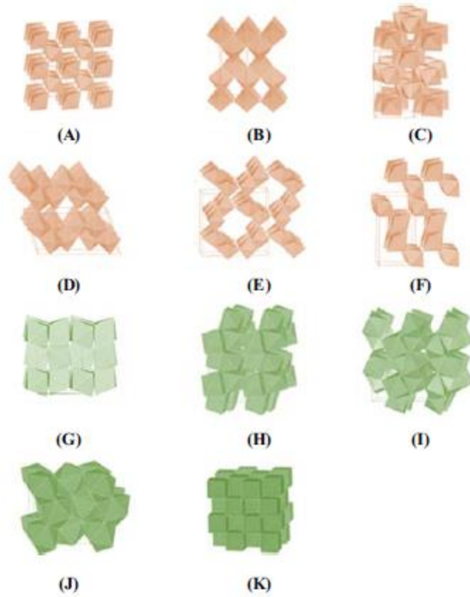
Şekil 2.2 Polihedron modellerde \text{TiO}_2 'nin 11 fazı: (A) rutil, (B) anataz, (C) brukit, (D) \text{TiO}_2(\text{B}) , (E) hollandit benzeri \text{TiO}_2(\text{H}) , (F) ramsdelit benzeri \text{TiO}_2(\text{R}) , (G) kolumbit benzeri \text{TiO}_2(\text{II}) , (H) baddeleyit benzeri, (I) \text{TiO}_2(\text{OD}) , (J) kotunit benzeri \text{TiO}_2(\text{OII}) ve (K) florit benzeri kübik fazlar (Parrino vd. 2021). Birim hücreler ince çizgiler ile gösterilmiştir.
