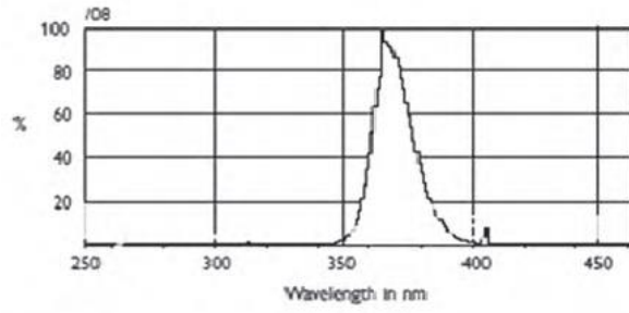
Şekil 3.3 UVA floresan lambasının (Philips, 8W) spektrumu.
