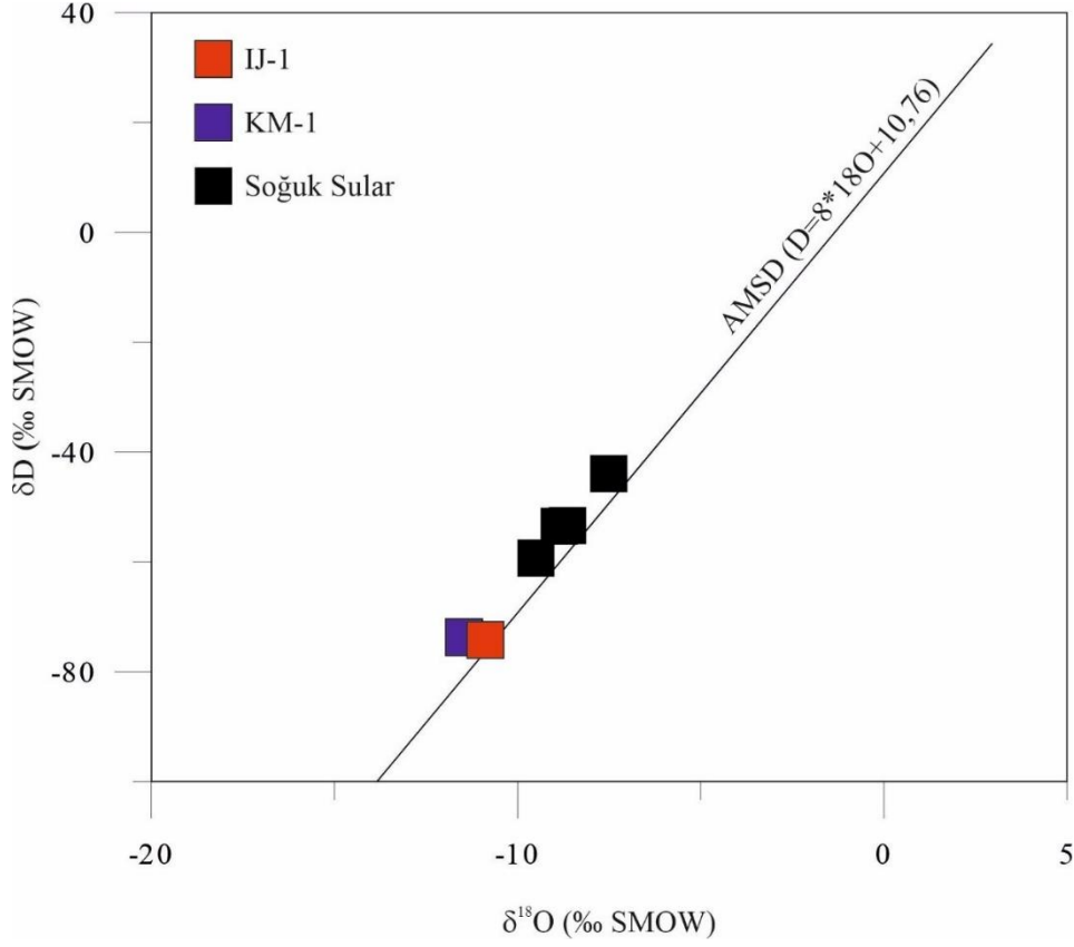
Şekil 7.1 Su örneklerinin ^{18}\text{O} -D diyagramındaki konumu.
