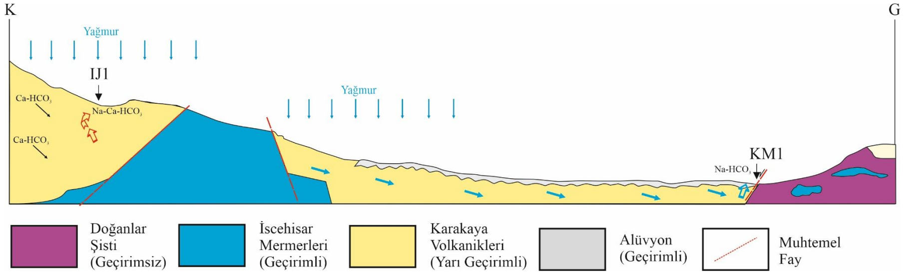
Şekil 5.5: İscehisar jeotermal sahasının kavramsal modeli (ölçeksiz).
