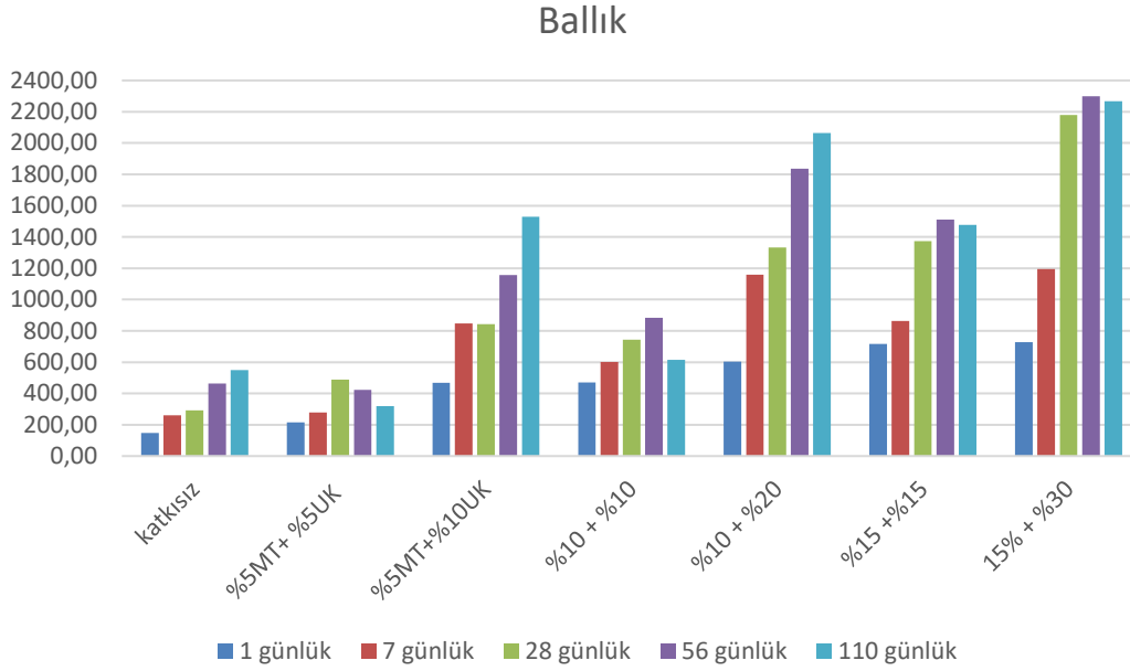
Şekil 4.6 Ballık numunesi eksenel basınç deney sonuçları.
