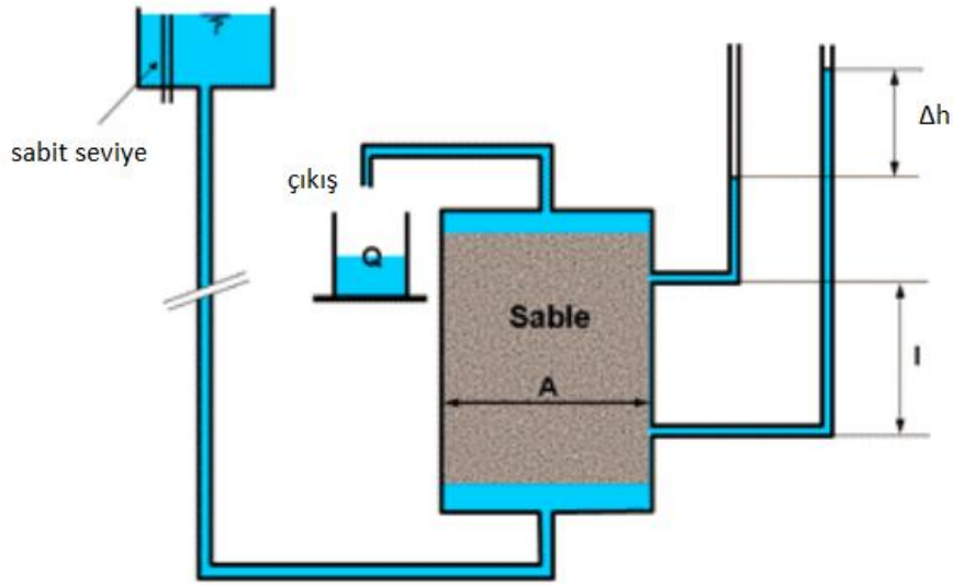
Şekil 3.7 Sabit seviyeli (İnt.Kyn. 4).
