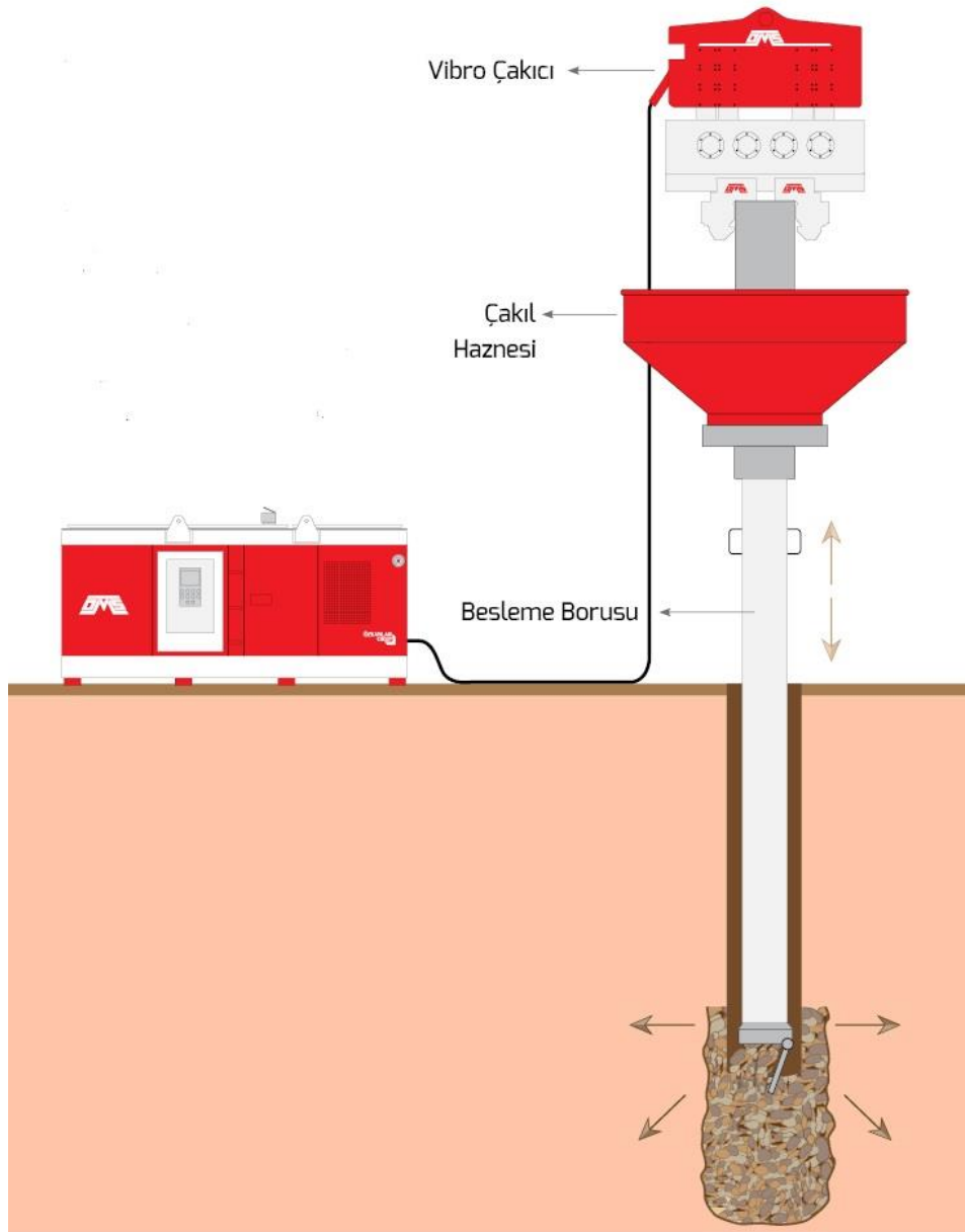
Şekil 2.2 Vibrokompaksiyon ekipmanı (İnt.Kyn. 1).
