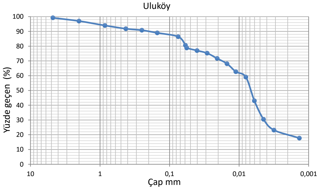
Şekil 3.1 Uluköy numunesinin granulometri grafiği.
