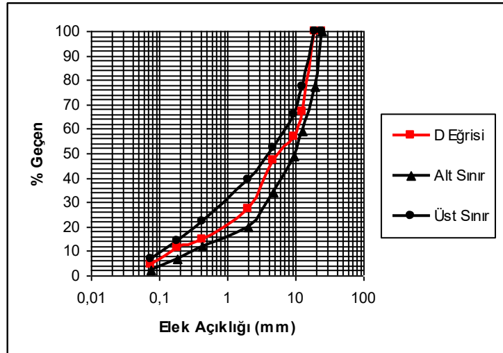
7.14 C Numunesine Ait Granülometri
