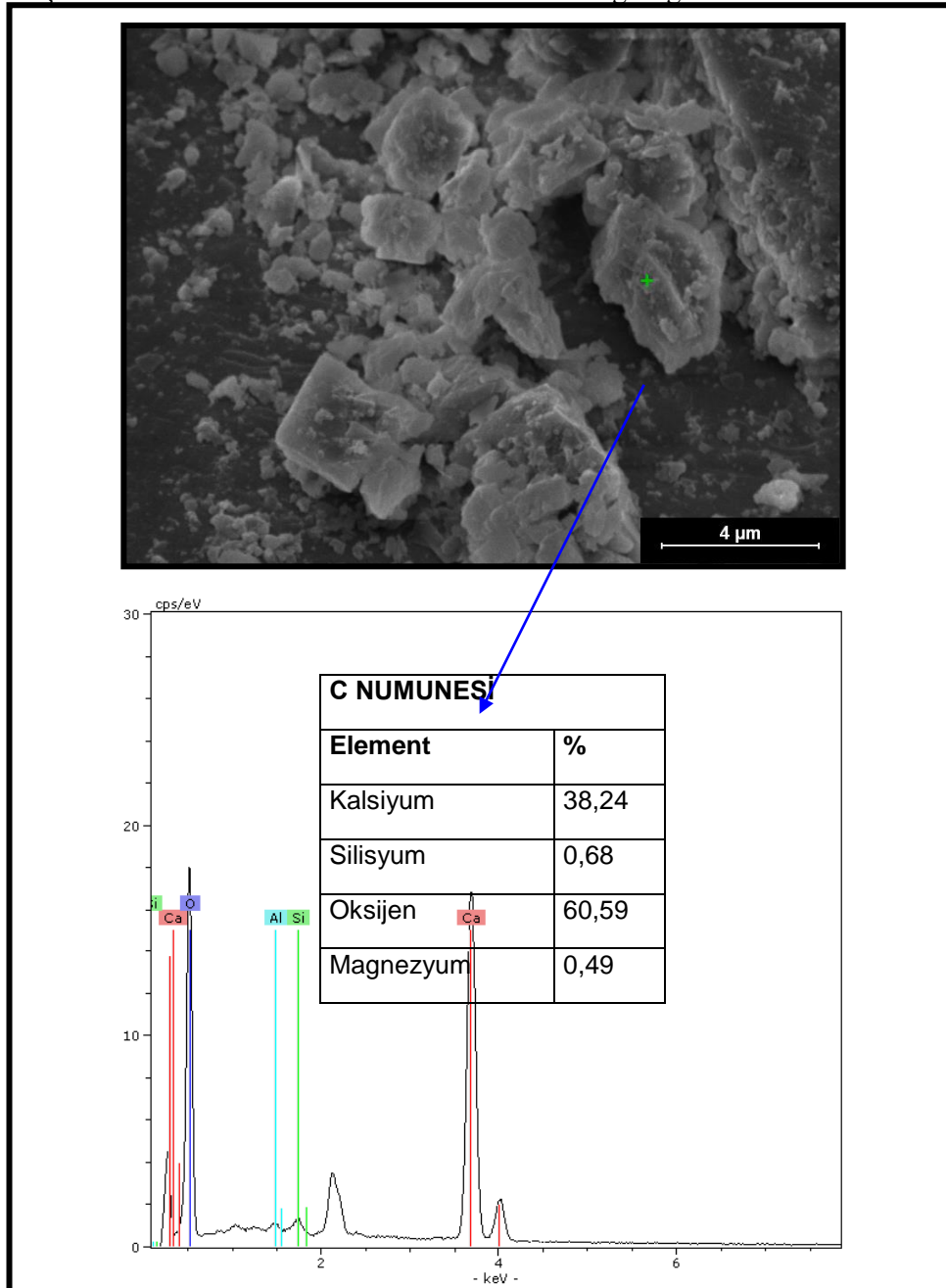
Şekil 7.10 C numunesinde kalsit kristalinin EDX grafiği ve EDX analiz sonucu.
