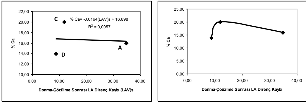
Şekil 7.25 % Ca ile (LAV) s arasındaki ilişki.
