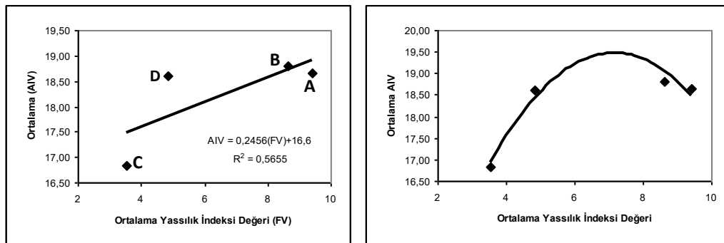
Şekil 7.28 Darbelenme Değeri ve Yassılık İndeksi Arasındaki İlişki.
