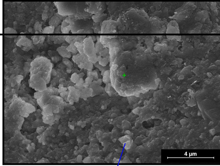
Şekil 7.9 numunesinde kristalinin grafığı ve EDX sonuçları.
