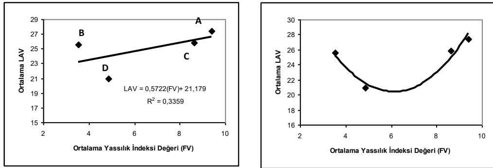
Şekil 7.27 Los Angeles Aşınma Kaybı ve Yassılık İndeksi Arasındaki İlişkiler.
