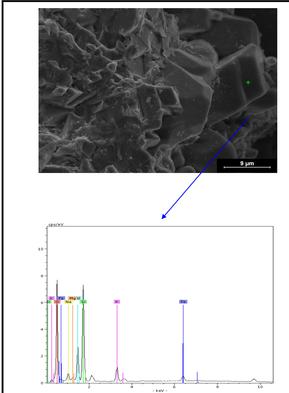
Şekil 7.3 B numunesinde feldspat kristalinin EDX grafiği ve EDX analiz sonucu.
