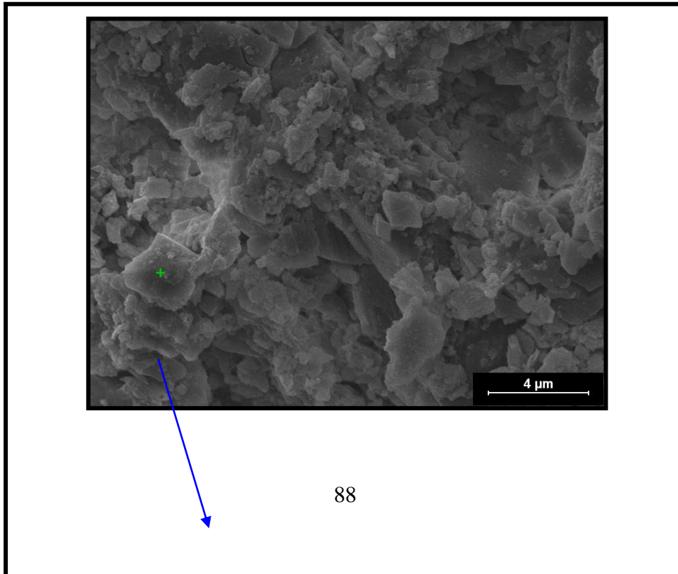
Şekil 7.8 Mikrokristalin kalsit kristalleri.
