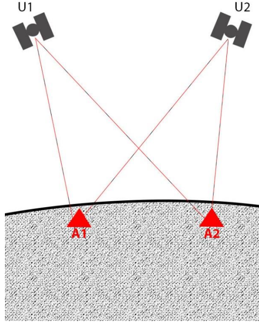
Şekil 3.2 Alıcılar arasında ikili fark gözlemleri.
