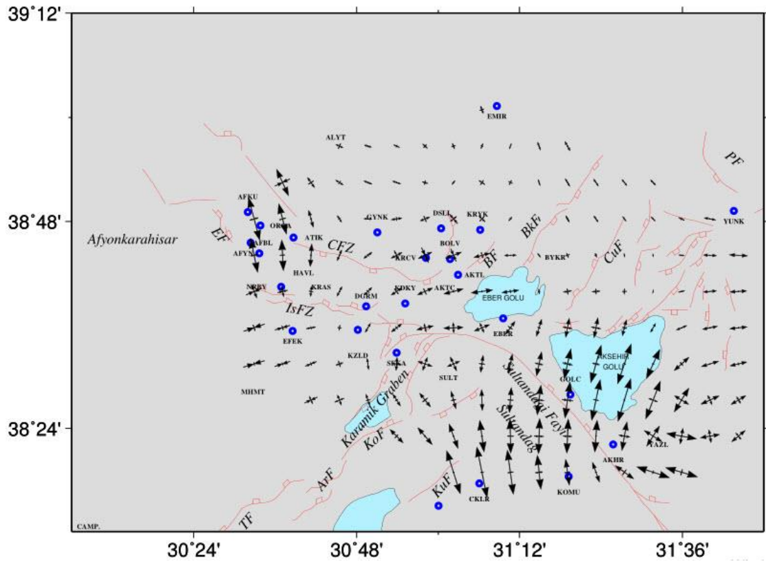
Şekil 6.5 Bölgenin yamulma alanı.
