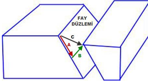
Şekil 2.6 Yanal atımlı fay şekli (Tiryakioğlu 2012).
