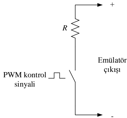
Şekil 3.2 Ayarlanabilir yük devresi prensip şeması.
