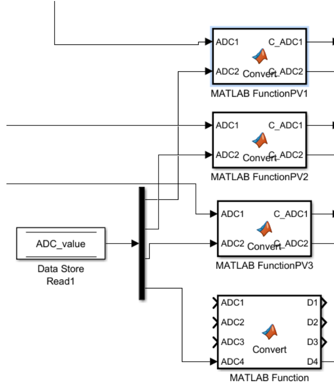
Şekil 3.17 ADC değerlerinin matematiksel fonksiyonlara giriş olarak uygulanması.
