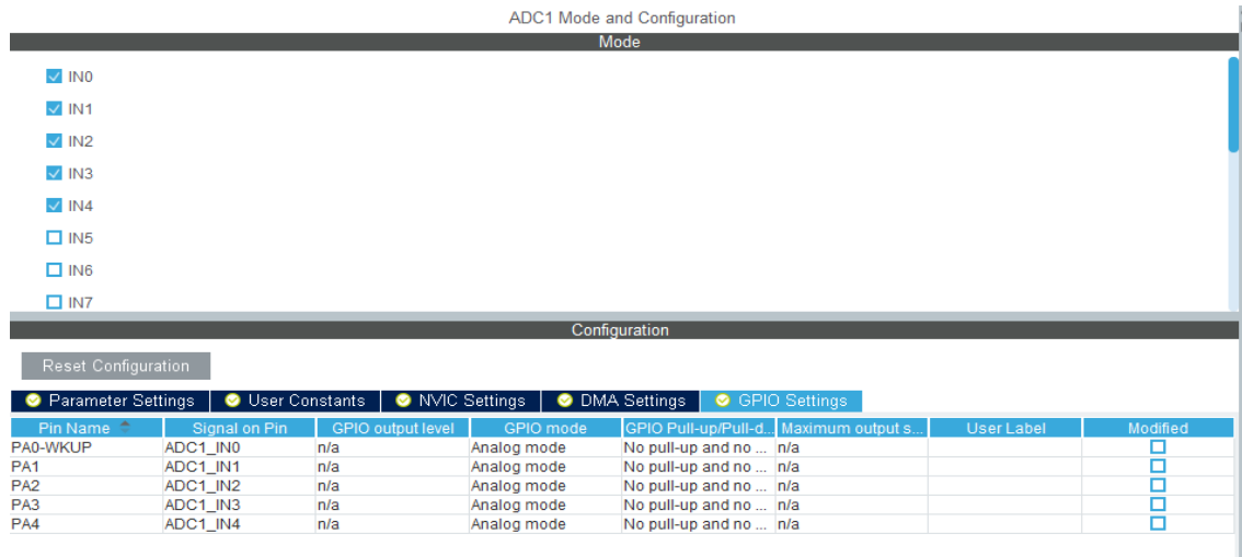
Şekil 3.6 ADC ayarları.
