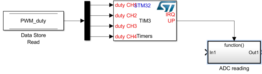
Şekil 3.21 PWM değerlerinin üretilmesi.
