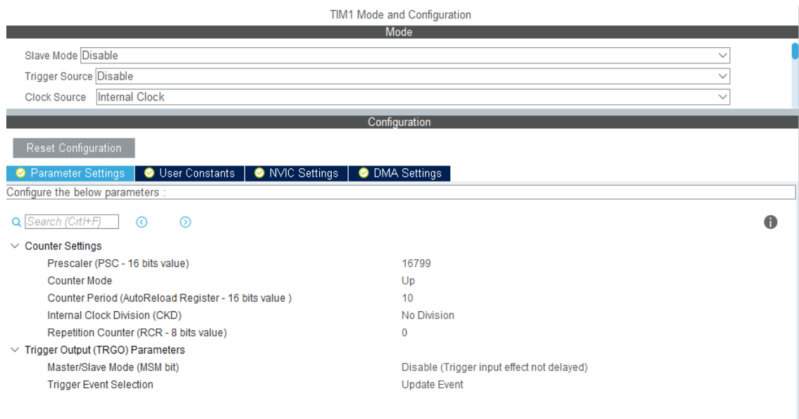
Şekil 3.7 TIMER 1 ayarları.
