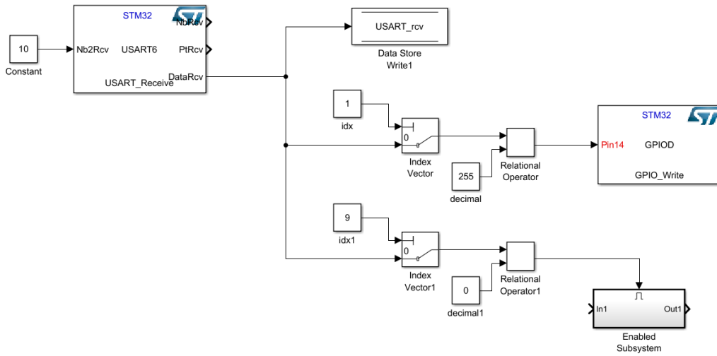
Şekil 3.26 USART veri alma bloklarının görünümü.
