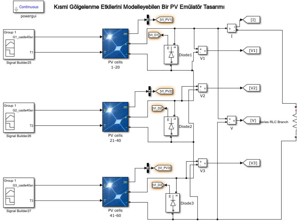
Şekil 3.31 Farklı senaryolarla PV modellerinin simüle edilmesi.
