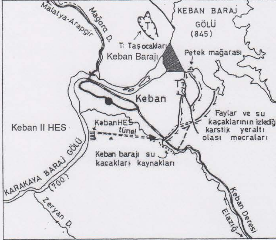
Şekil 3: Keban baraj gölünde meydana gelen kaçak alanları. Su kaçakları ve yapılan ek masraflar baraj yeri seçilirken paleokarst ve karst morfolojisi ile ilgili çalışmaların önemini ortaya koymuştur.
