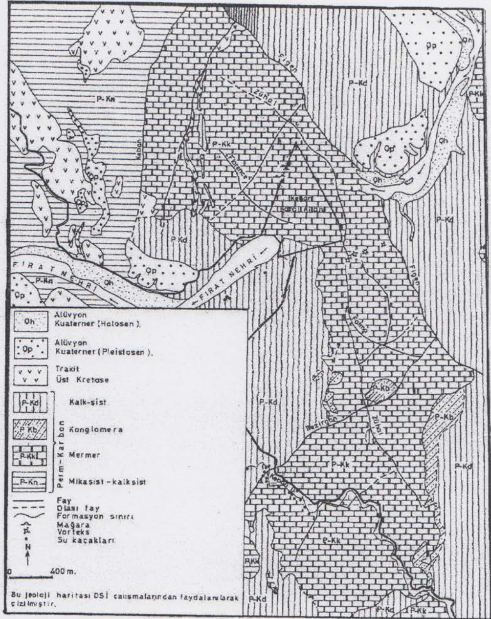
Şekil 1: Keban baraj inşaat alanı ve yakın çevresinin jeoloji haritası
