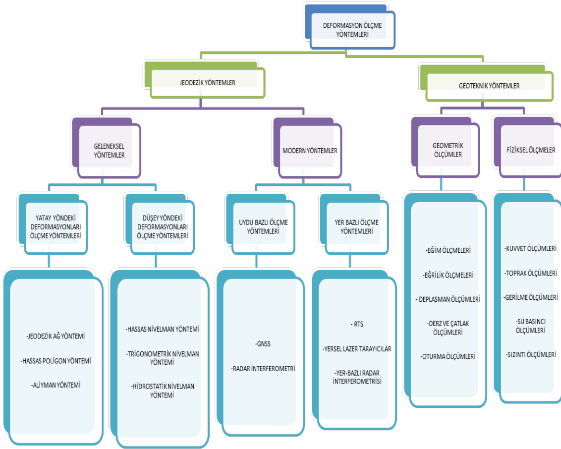
Şekil 4.2 Deformasyon ölçme yöntemleri.
