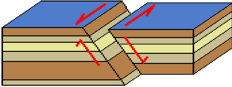
Şekil 2.4 Oblik (yanal) atımlı fay türleri (İnt. Kyn. 2).
