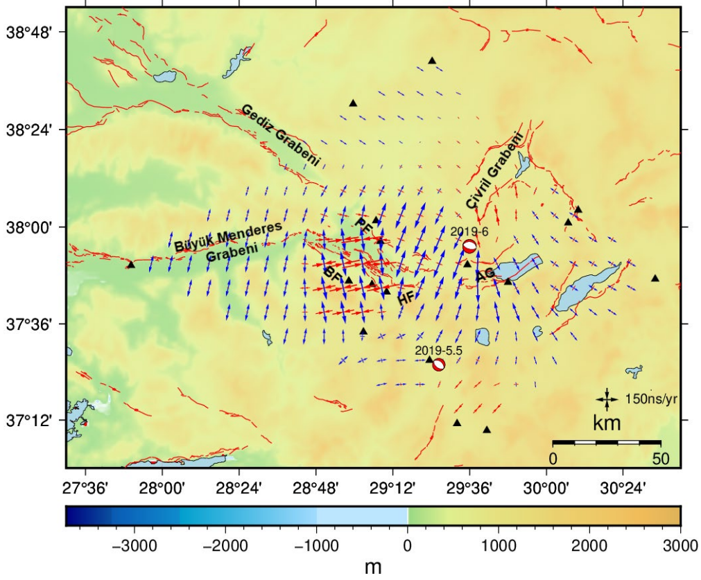
Şekil 5.5 Gerinim alanı ve Bozkurt (Mw:6.0), Acıpayam (Mw:5.5) deprem çözümleri.
